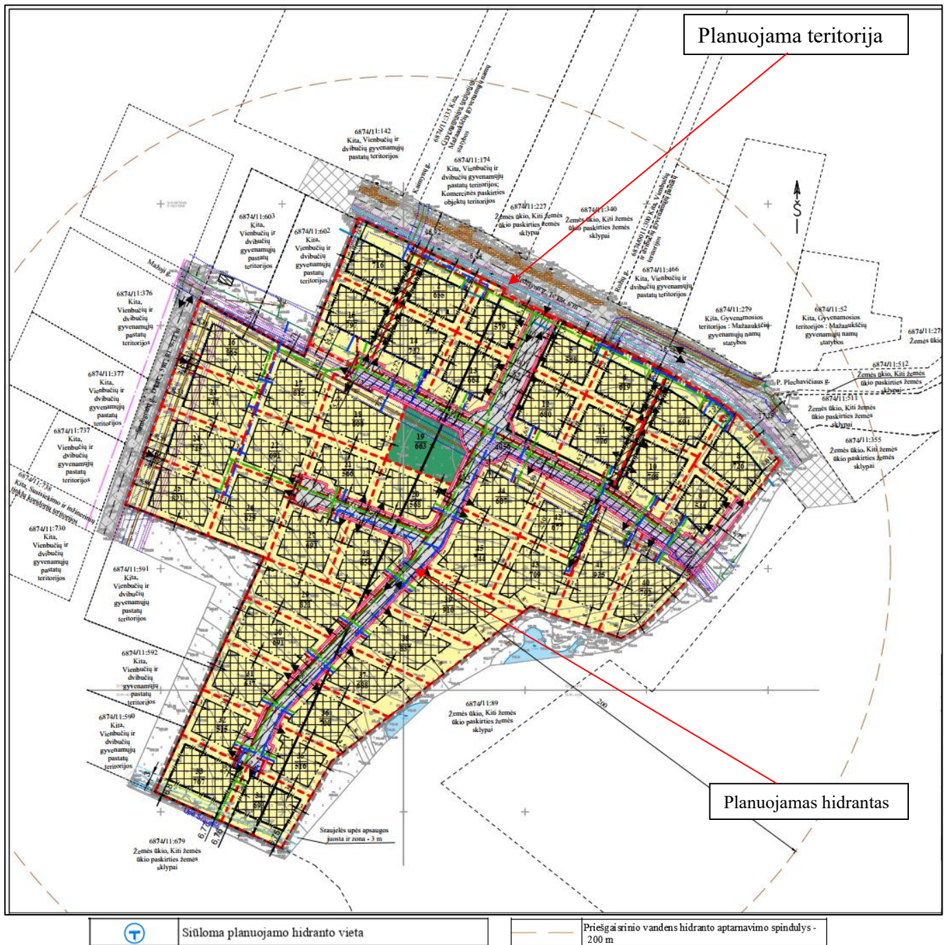
4 pav. Ištrauka iš galimų teritorijos aprūpinimo inžineriniais tinklais ir susisiekimo komunikacijomis būdų schemos brėžinio
