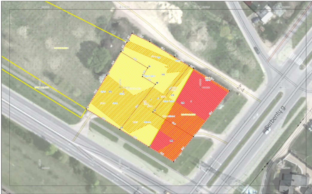
Sprendinių brėžinys (Žemės sklypų formavimo projektas) 1 Lapas M 1:500
