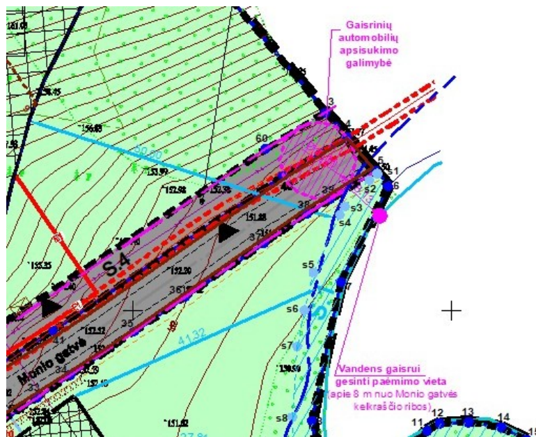
18 pav. Gaisrinių mašinų apsisukimo galimybė ir vandens paėmimo vieta
