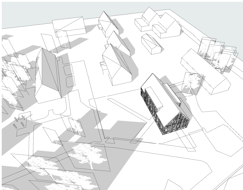
Projektuojamo pastato šešėlis kovo 22 d. ir rugsėjo 22 d. 14 val. :
