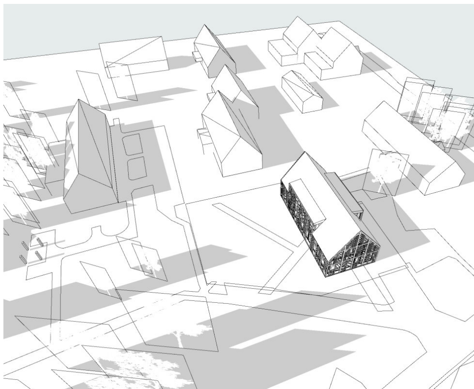
Projektuojamo pastato šešėlis kovo 22 d. ir rugsėjo 22 d. 14 val. :
